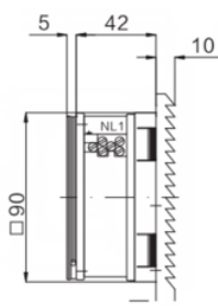
侧视图(入口) Side View(Inlet)
