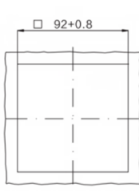
安装开孔图 Cut-out
